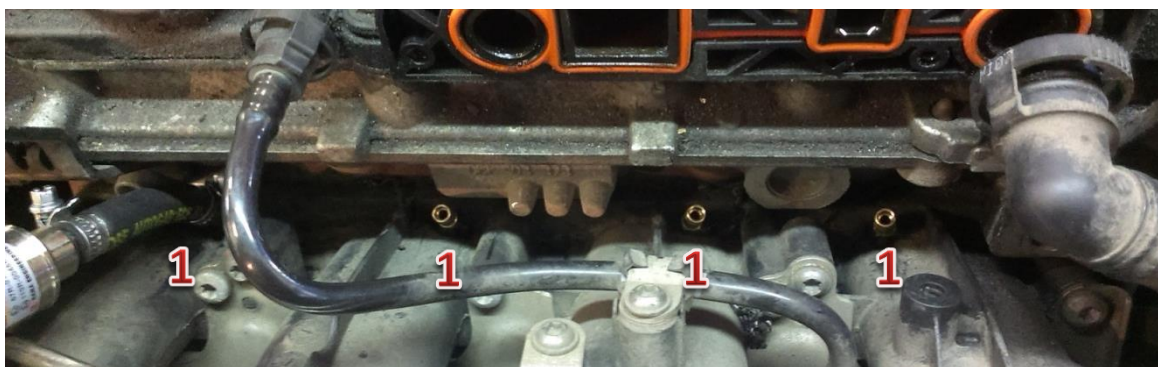
1-dysze wtryskiwaczy gazu/gas injector nozzles
