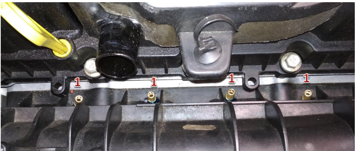
1-dysze wtryskiwaczy gazu/gas injector nozzles
