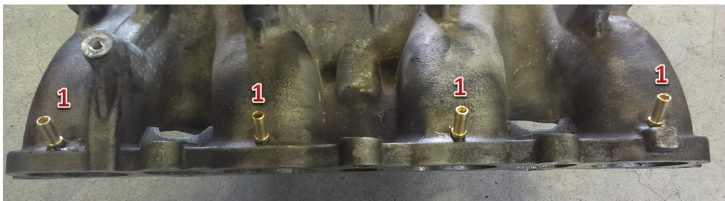
1-dysze wtryskiwaczy gazu/gas injector nozzles,
