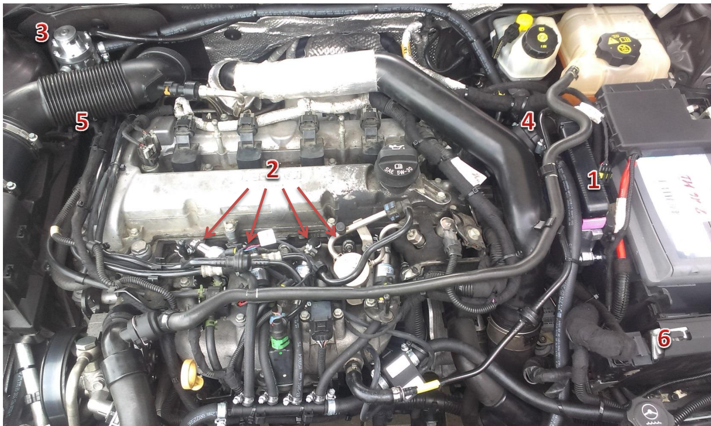
1-sterownik/ECU Zenit Direct 2-wtryskiwacze gazu/gas injectors, 3-reduktor/reducer, 4-filtr fazy lotnej/gas phase filter, 5-elektrozawór z filtrem fazy ciekłej/electrovalve with liquid gas phase filter, 6 - petrol ECU
