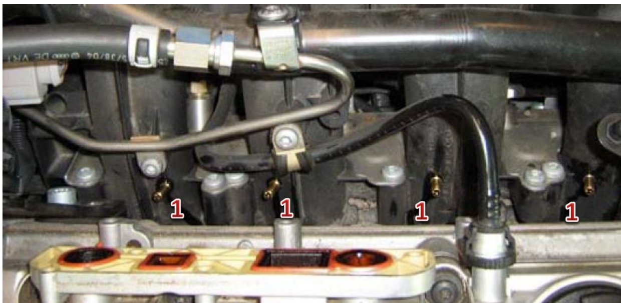
1-dysze wtryskiwaczy gazu/gas injector nozzles
