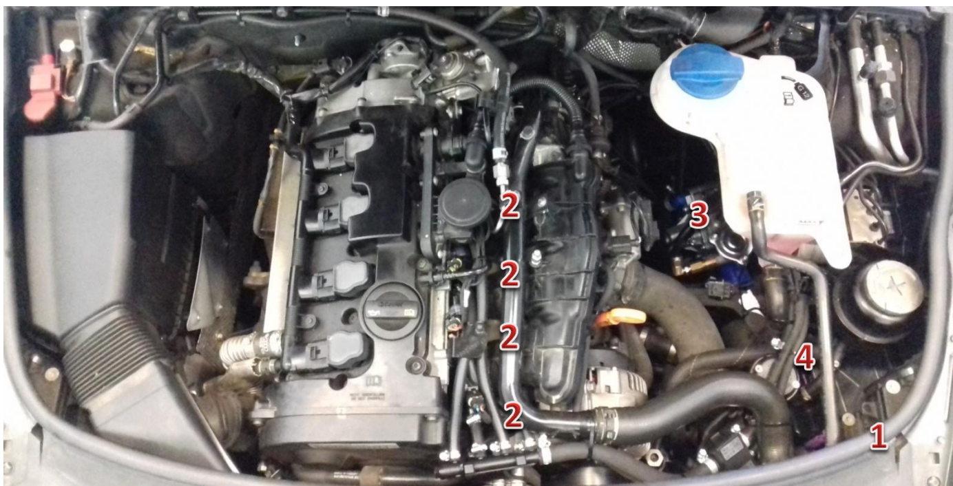
1-sterownik/ECU Zenit Direct, 2-wtryskiwacze gazu/gas injectors, 3-reduktor/reducer, 4-filtr fazy lotnej/gas phase filter
