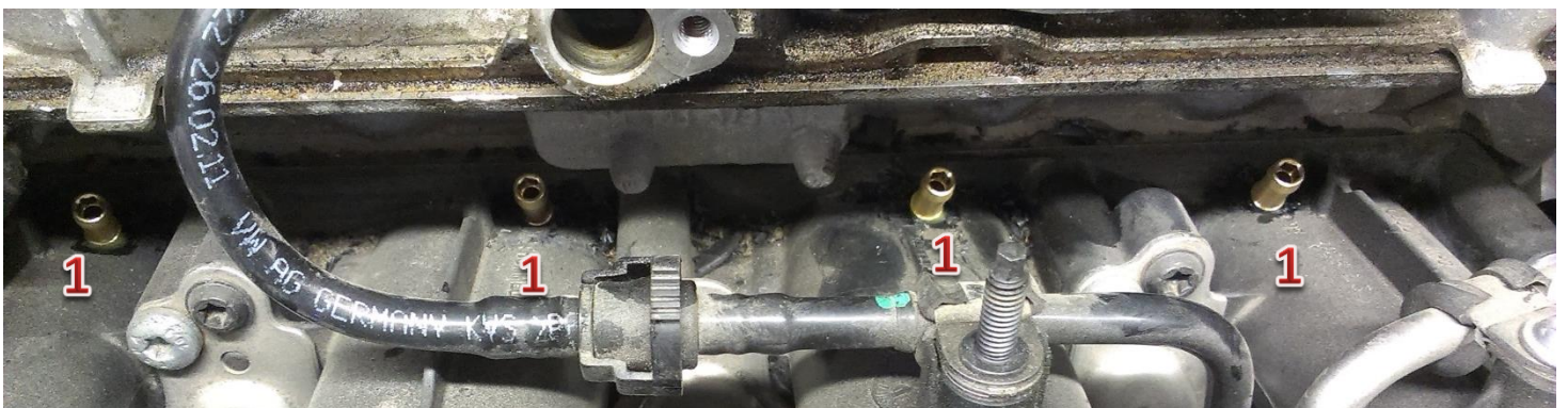
1-dysze wtryskiwaczy gazu/gas injector nozzles
