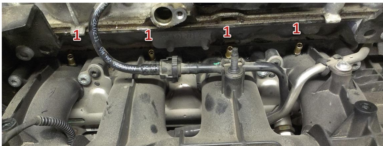
1-dysze wtryskiwaczy gazu/gas injector nozzles
