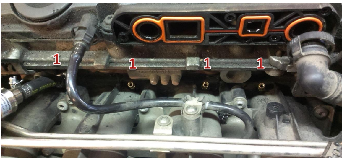
1-dysze wtryskiwaczy gazu/gas injector nozzles
