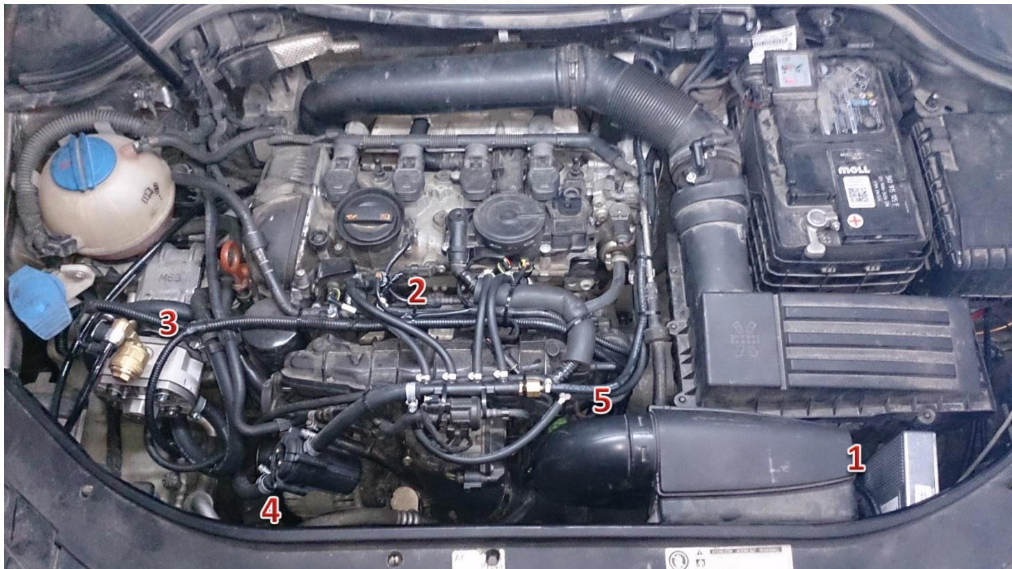
1-sterownik/ECU Zenit Direct, 2-wtryskiwacze gazu/gas injectors, 3-reduktor/reducer, elektrozawór z filtrem fazy ciekłej/electrovalve with liquid gas phase filter, 4-filtr fazy lotnej/gas phase filter, 5- króciec podciśnienia/vaccum nozzle
